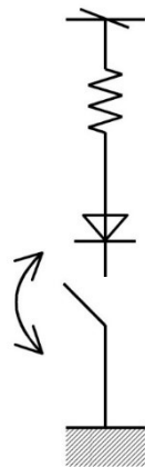
図 3. 回路図
